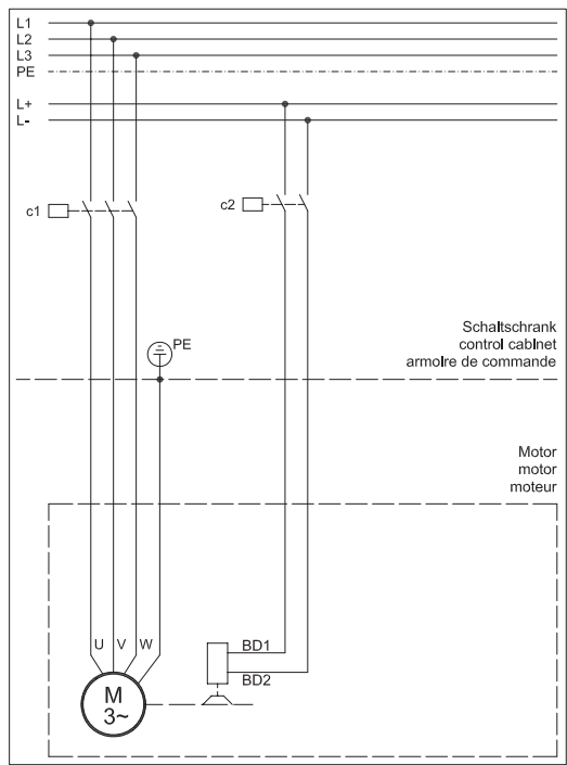
Bild 4: Direkte Gleichspannungsversorgung aus einem Steuernetz
