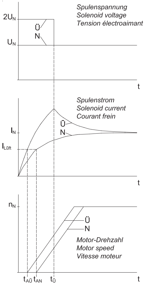
Bild 2: Prinzipieller Verlauf der Spulenspannung, des Spulenstroms und der Motordrehzahl bei Normalerregung (N) und Übererregung (Ü).
