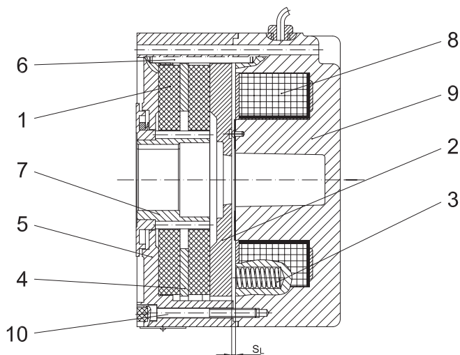
Bild 1: Zweischeiben-Federdruckbremse der Reihe Z..
