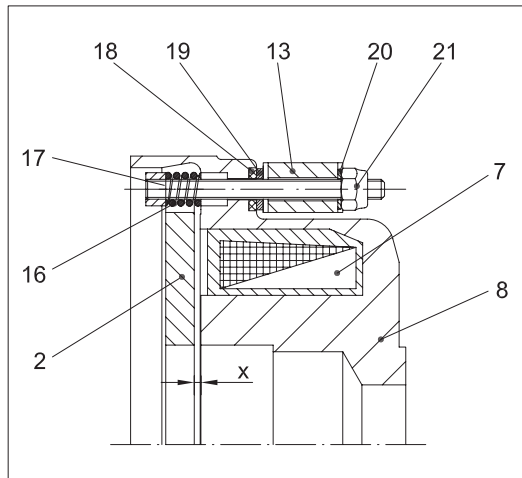
Bild 12: Montage der Handlüftung
