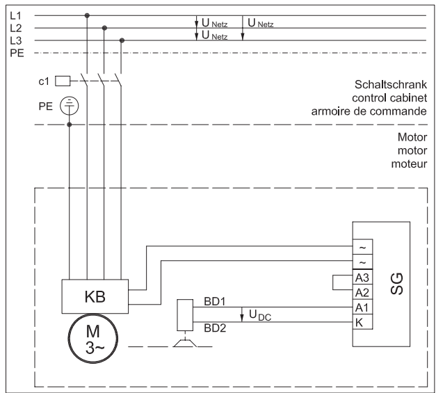
Bild 5: Wechselstromseitige Abschaltung → Klemme A2 und A3 gebrückt
