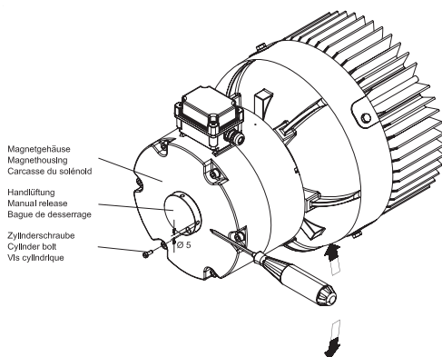
Bild 12: Bremse - Typen E../Z..075 und Z..100 - mit arretierbarer Handlüftung Es darf nur die Original-Zylinderschraube verwendet werden, da ansonsten die Bremse in ihrer Funktion gestört werden kann (Schraubenlänge beachten). Der Lüftring dient nicht zur Nachstellung des Luftspalts !
