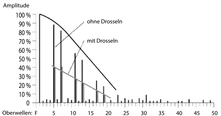
Reduzierung der Netzurückwirkungen bei Frequenzumrichtern.
